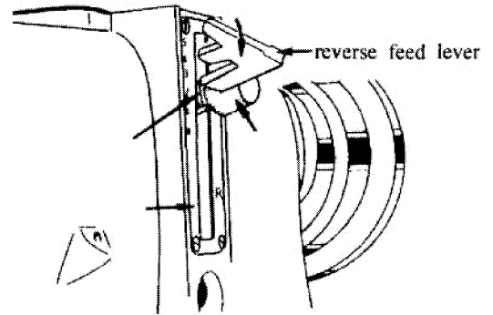
Reverse feed lever Рычаг обратной подачи
